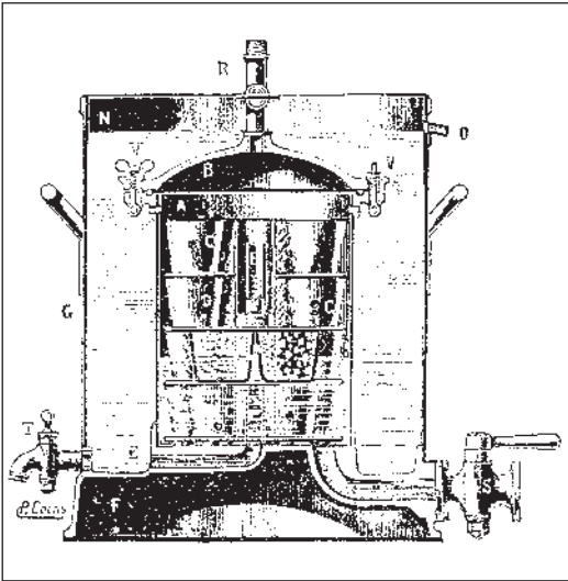
2. ábra: A készülék belső felépítése (VeML V. 173. b VII/597 1900)
