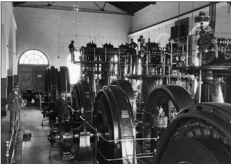
A villanytelep gépháza. Forrás: LDM 7653
