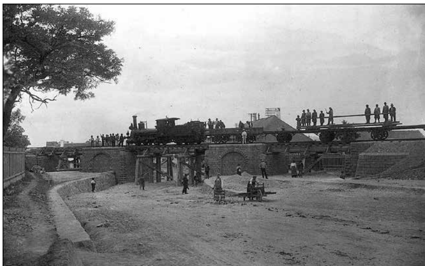
Veszprémi áthidalás a Palotai útról nézve
