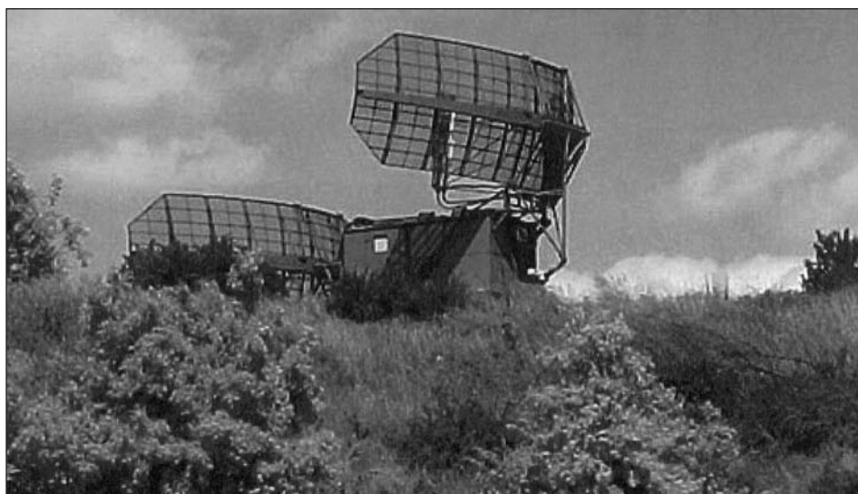
P-37 „Bar Lock” rádiólokátor (MN54. Veszprém Légtérellenőrző Ezred)
