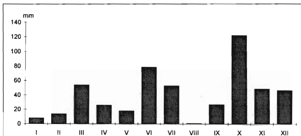
Havi csapadékösszegek, 1992
