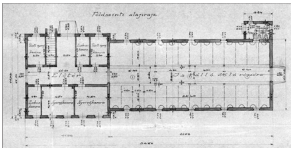
A régi főépület alaprajza 1926-ban
