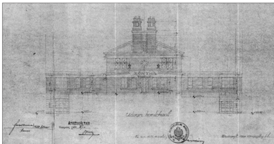
Gazdasági épület és konyha udvari homlokzata 1930-ban
