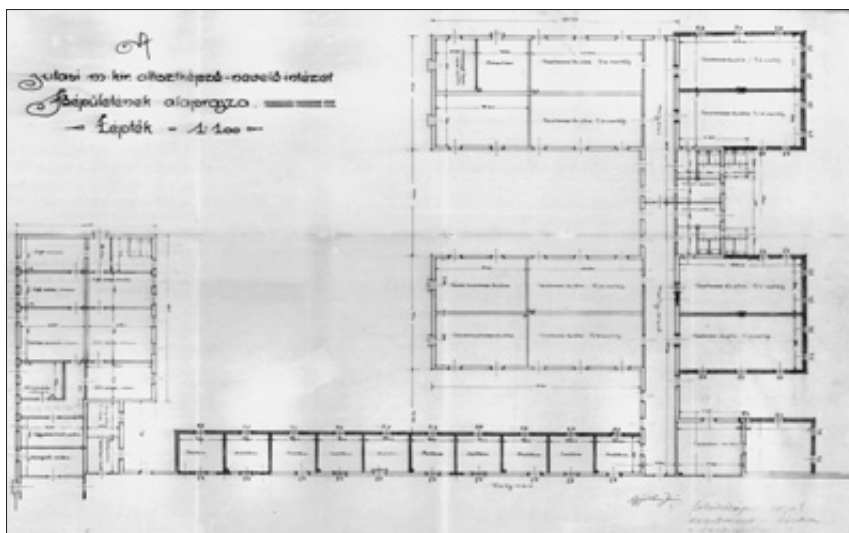
A régi főépület alaprajza 1926-ban
