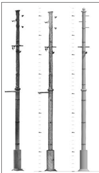
Betonkorróziós károsodások az oszlopon
