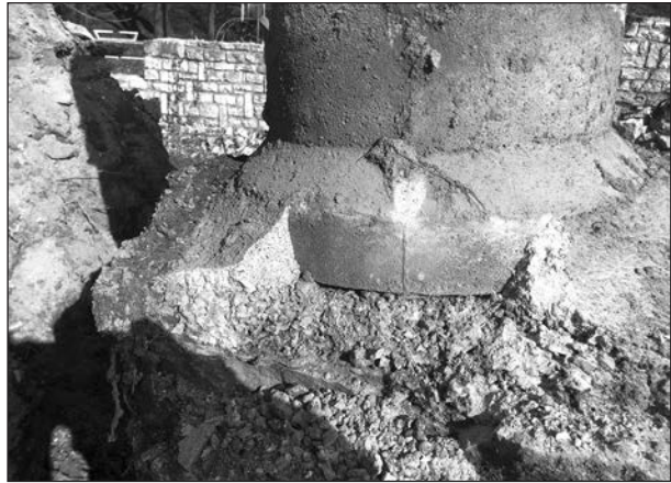
Kiemelt oszlop alapozása
