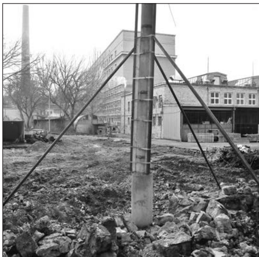
Ideiglenes megtámasztások
